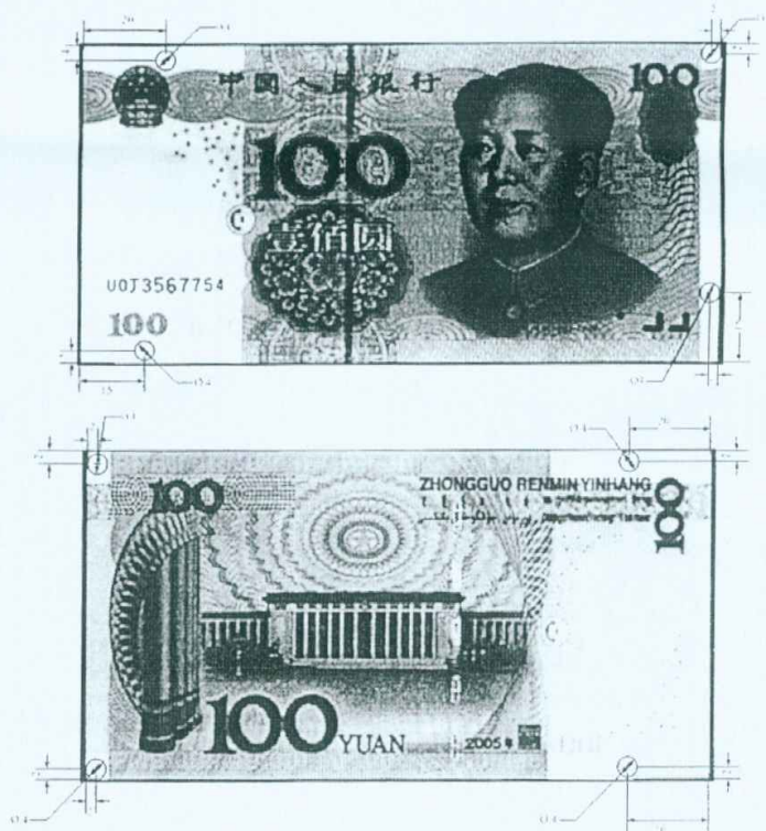
图A.1 壹佰圆检测采样点 (单位: mm)
